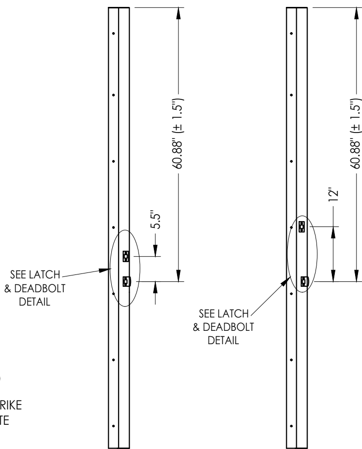
STRIKE JAMB
